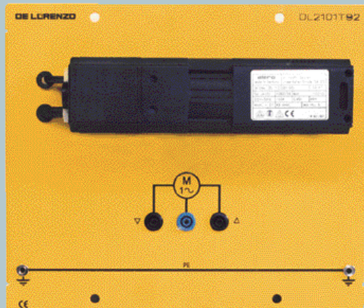
DL 2101T92 MOTEUR POUR STORE VENETIENS Moteur pour rideaux de type vénitiens avec fin de course et protection thermique intérieurs. Possibilité de régulations de la position oblique des lamelles. Caractéristiques techniques: Alimentations : 230V, 50-60Hz Courrant nominal : 0.25 A environ
